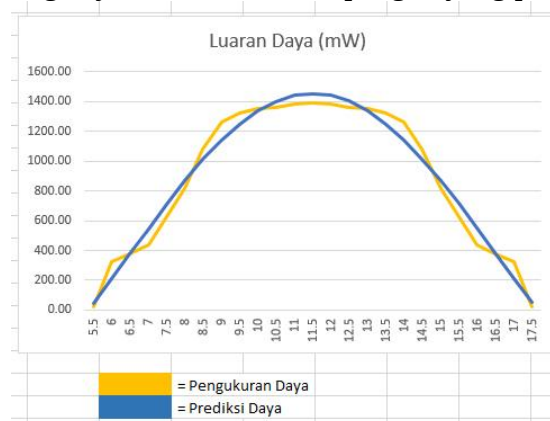
Gambar 4. Grafik Hasil Prediksi Pengukuran Daya
