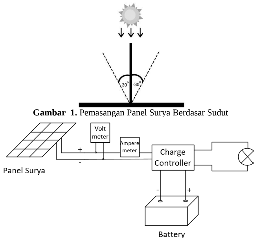
Gambar 2. Skematik Pemasangan Percobaan Pengukuran Luar Panel Surya
