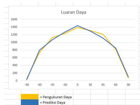
Gambar 3. Grafik Hasil Prediksi Dan Pengukuran Daya
